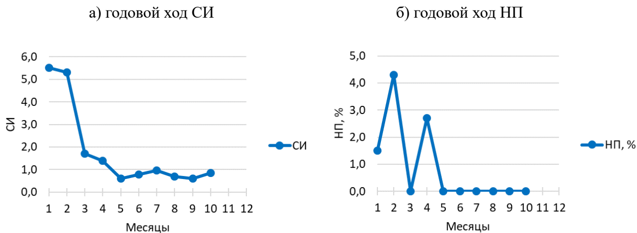
Рис. 16 — Годовой ход СИ и НП
